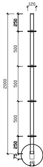
GIÁO RINGLOCK L=2000mmx2.5mm
