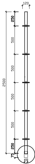
GIÁO RINGLOCK L=2500mmx2.5mm
