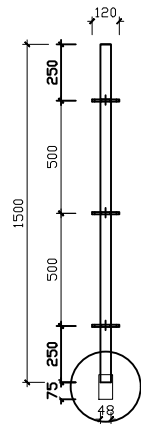
GIÁO RINGLOCK L=1500mmx2.5mm
