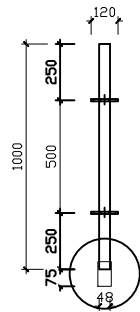
CHI TIẾT ỚNG NỐI TL 1-2 ống nối hàn trực tiếp vào đuôi cây giáo
