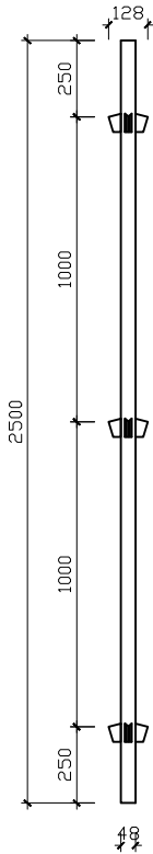
GIÁO NÊM L=2500mm
