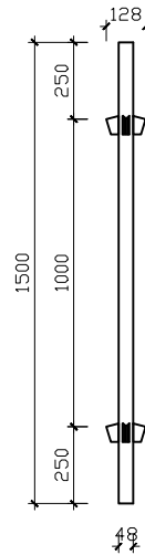
GIÁO NÊM L=1500mm
